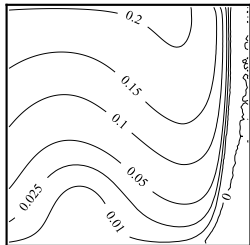
(d) (\nabla \cdot \sigma)_u Wachs.
