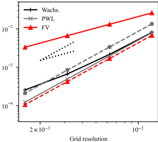
(b) (\nabla \cdot \sigma)_v
