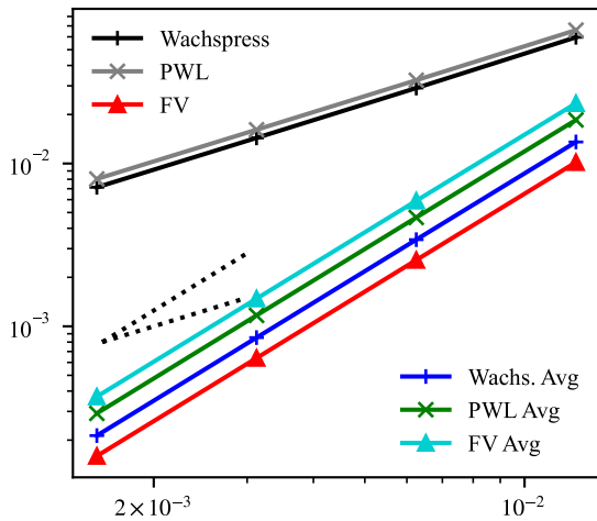
(d) Hex. \partial f/\partial y
