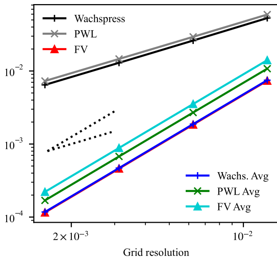
(d) Hex. \partial f/\partial y
