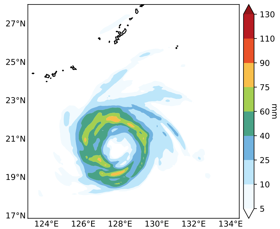
(d) Grell 3D Ensemble (cu = 5)
