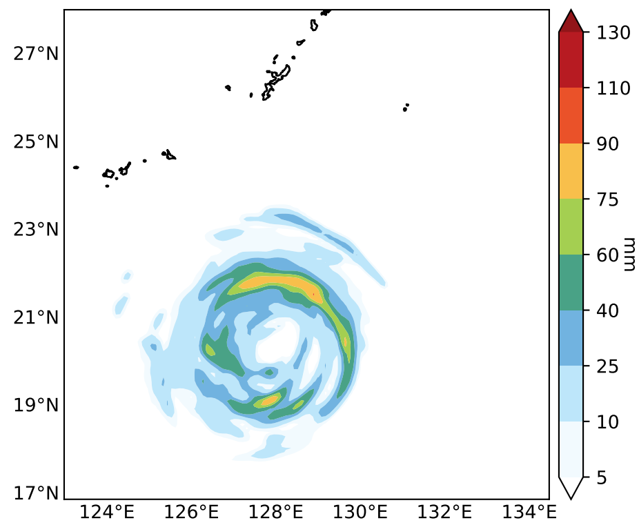
(a) No cu scheme (cu = 0)
