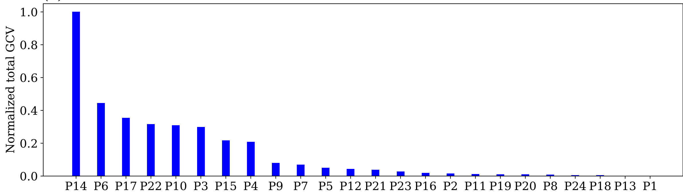
(b) MARS
