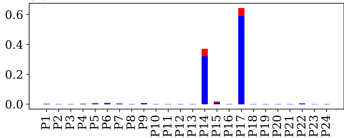
(d) RAIN
