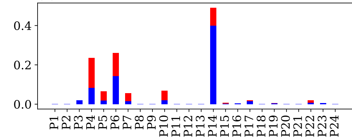
(e) PBLH
