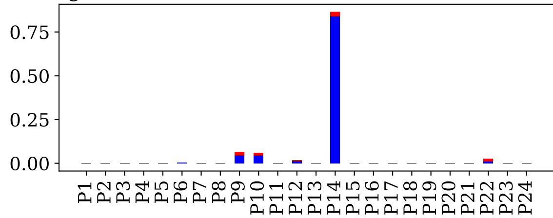
(g) DSWRF
