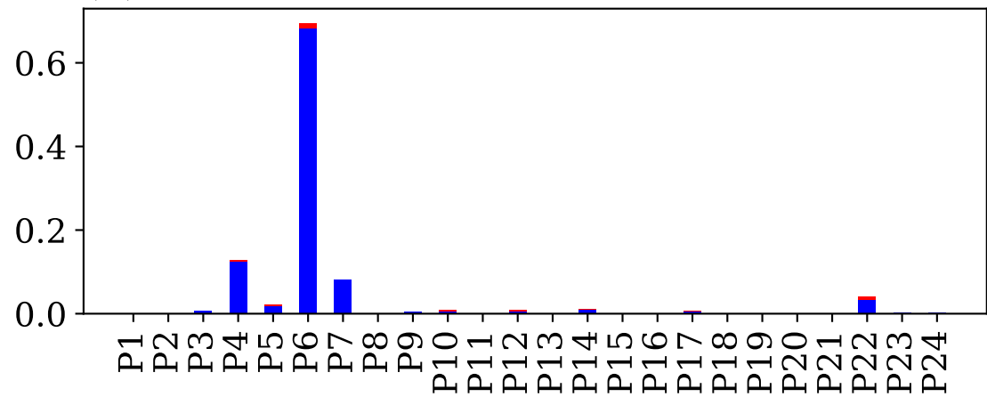
(f) OLR
