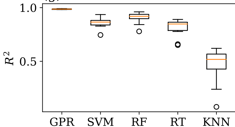
(g) DSWRF
