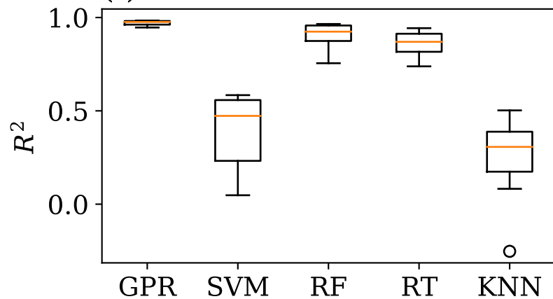
(f) OLR
