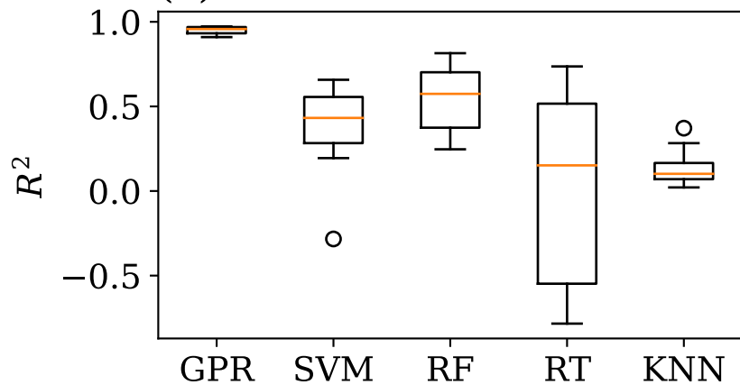
(e) PBLH
