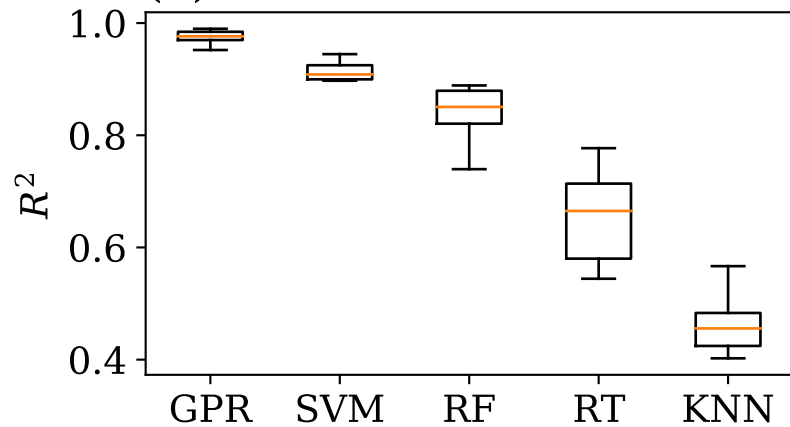
(d) RAIN
