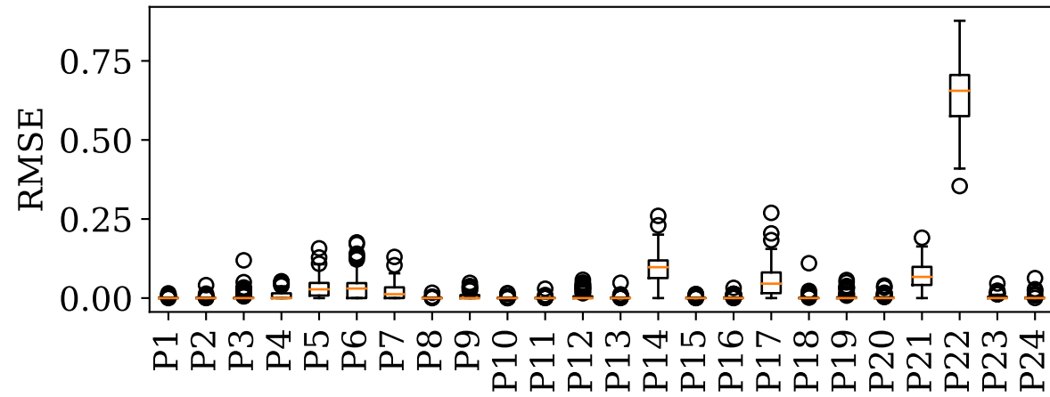
(g) DSWRF
