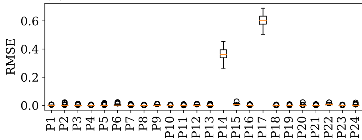
(d) RAIN
