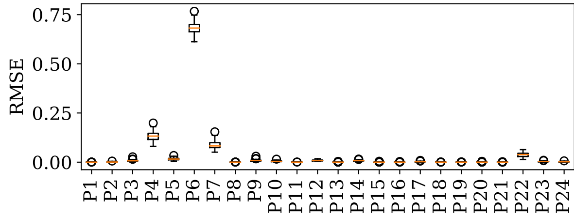
(f) OLR
