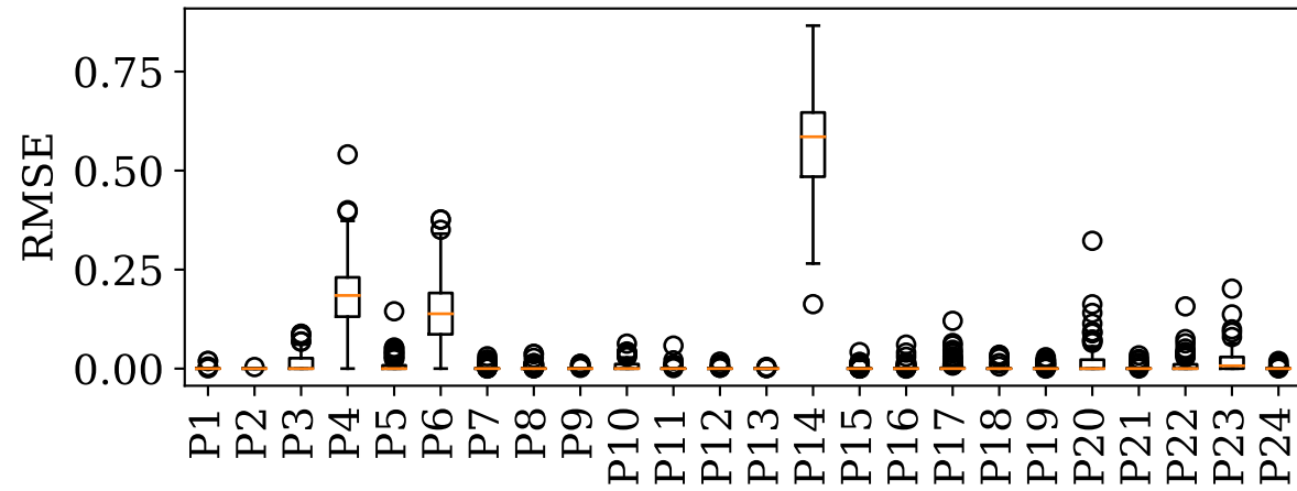
(e) PBLH
