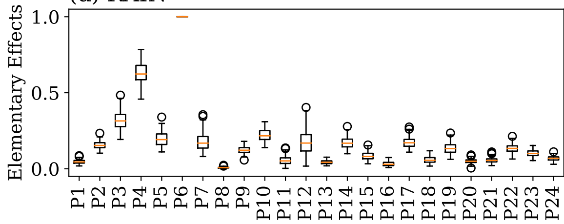
(f) OLR
