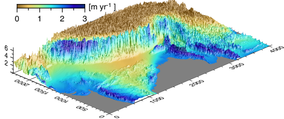
(d) Precipitation WorldClim2.1
