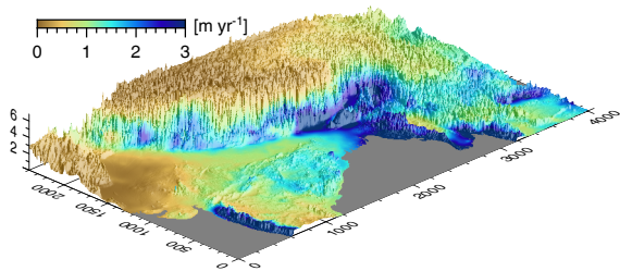
(d) Precipitation WorldClim2.1
