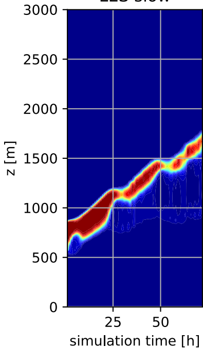
LES slow
