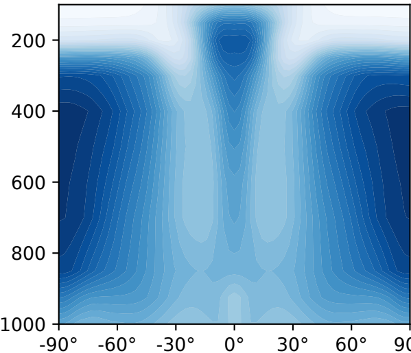
(d) Flex-UM slab ocean: RH
