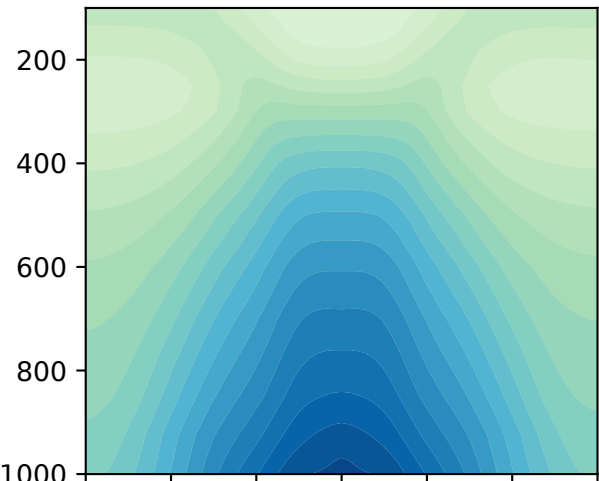
(d) Flex-UM slab ocean: RH
