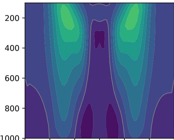
(d) Flex-UM fixed SST: \Psi
