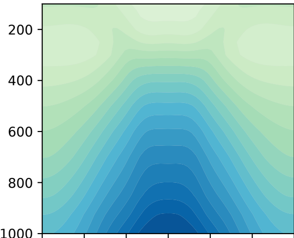
(d) Flex-UM fixed SST: RH
