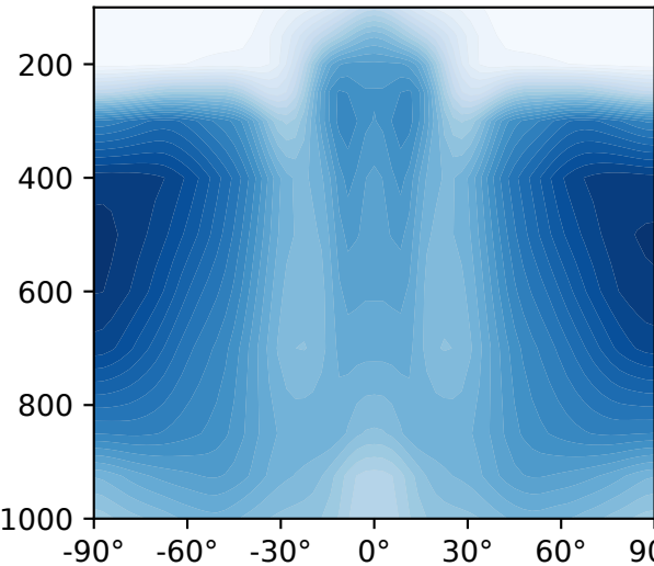
(d) Flex-UM fixed SST: RH
