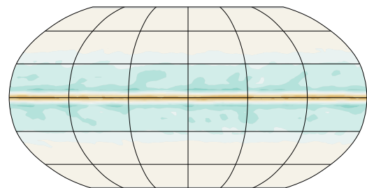
(c) Flex-UM - Isca: P
