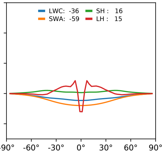
(f) Flex-UM - Isca: budget
