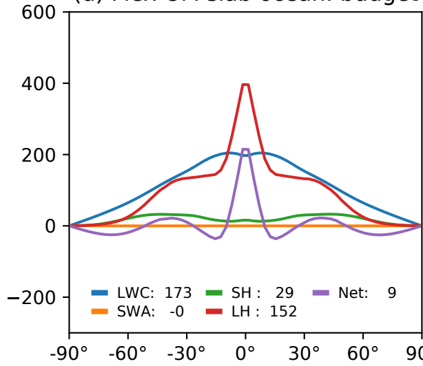
(d) Flex-UM slab ocean: budget
