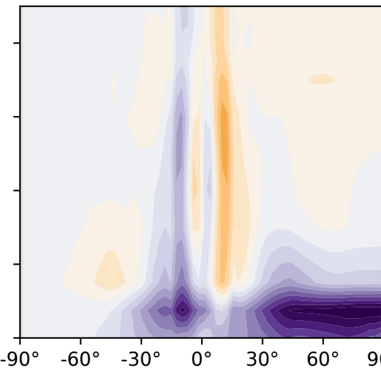
(f) Flex-UM - Isca: \Psi
