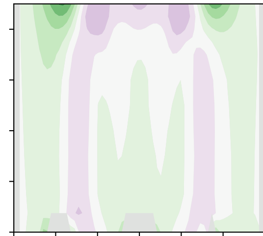
(f) Flex-UM - Isca: \Psi
