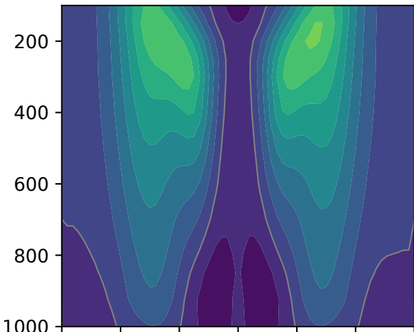
(d) Flex-UM slab ocean: \Psi
