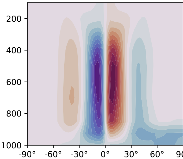
(d) Flex-UM slab ocean: \Psi
