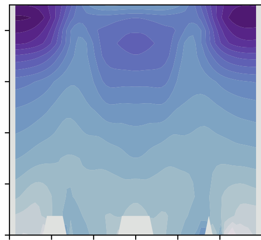
(f) Flex-UM - Isca: RH
