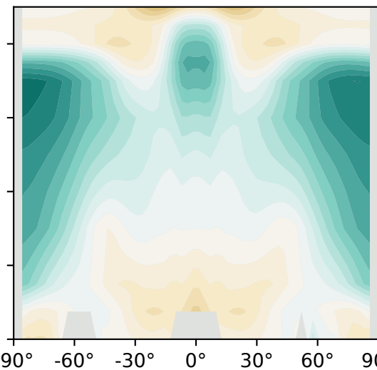
(f) Flex-UM - Isca: RH
