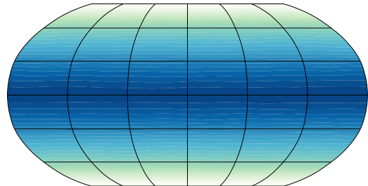
(d) GA7.0 Slab ocean: SST
