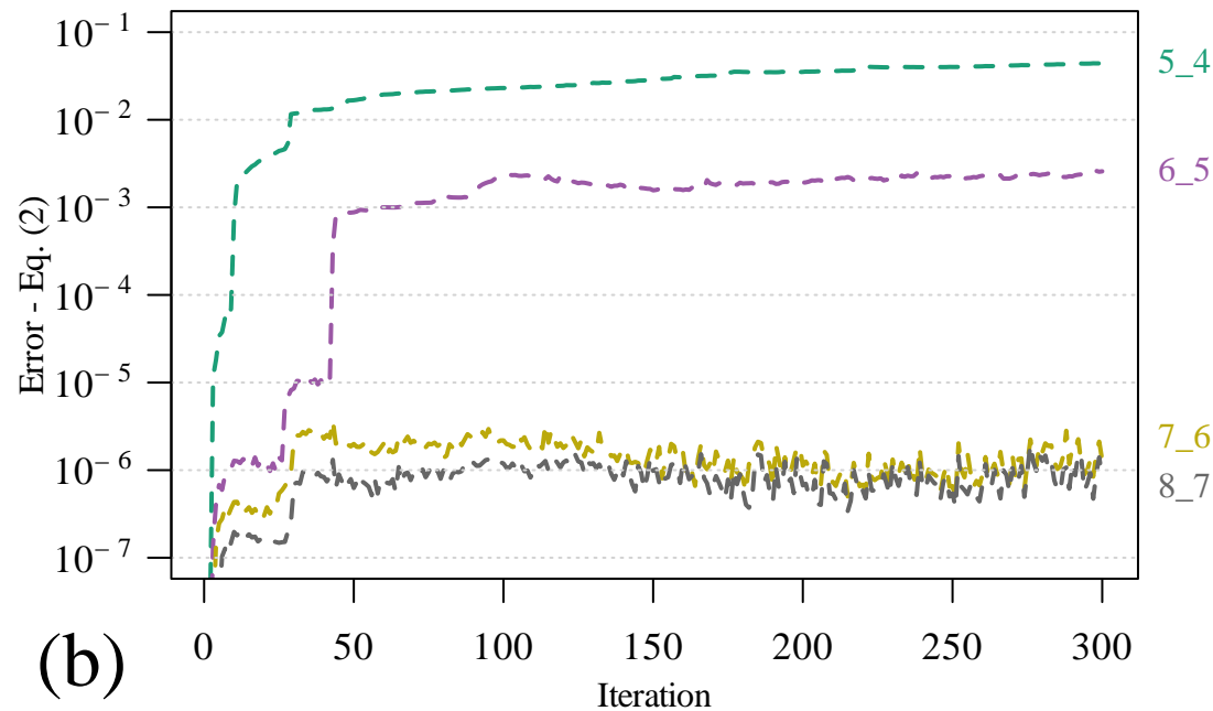
Hash on raw values
