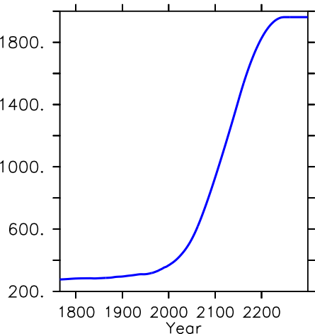
Atmos. CO 2 (ppm)
