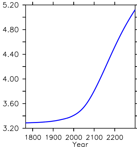
Ave. Ocean Temperature (°C)
