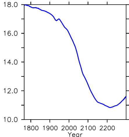
Maximum NH MOC (Sv)
