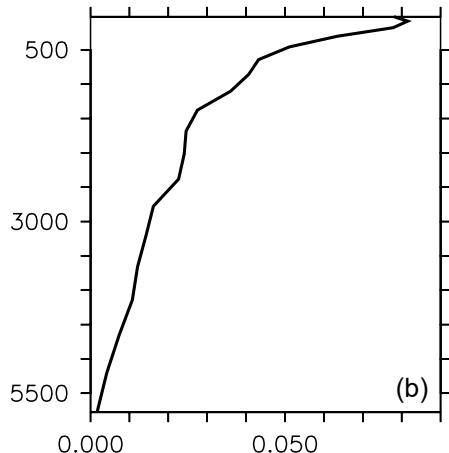
Opal Diss. ( \text{Tmol Si m}^{-1} \text{yr}^{-1} )
