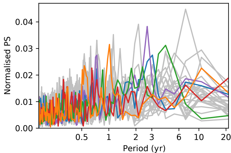
(f) SAM over 1958-2014
