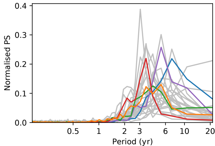
(d) NAM over 1958-2014
