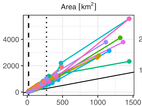
(d) WRF + TITAN (P3)
