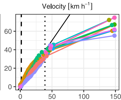
(f) WRF + TITAN (P3)
