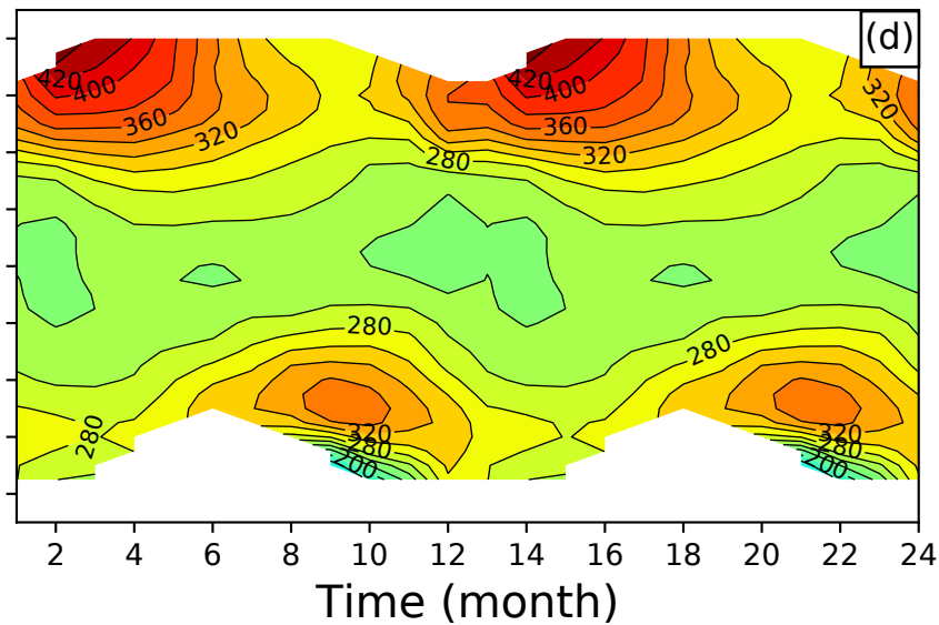
SBUV
