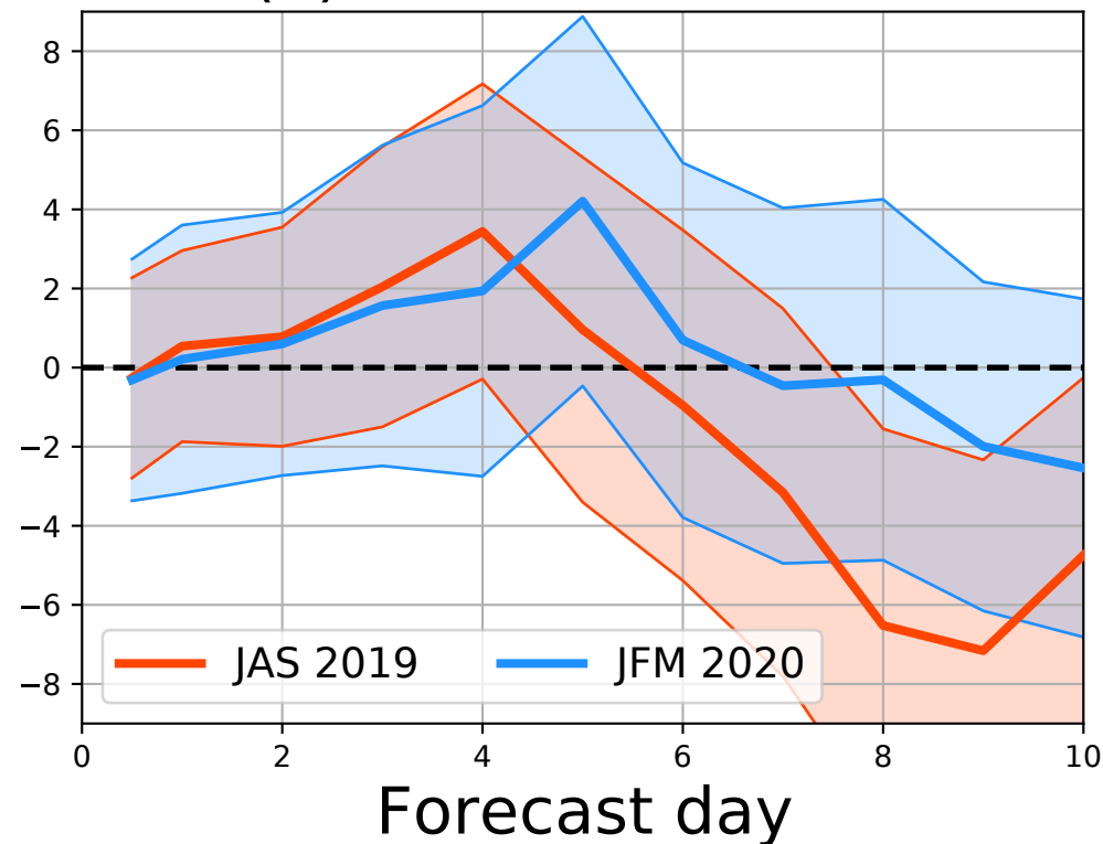
(d) Z: Arctic 500 hPa
