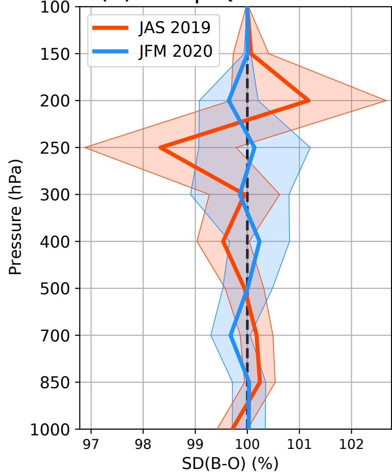
(d) Temp Q - N. Hemis.
