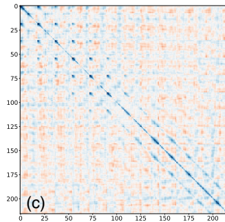
M1QN3
