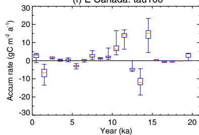
(f) E Canada: tau100
