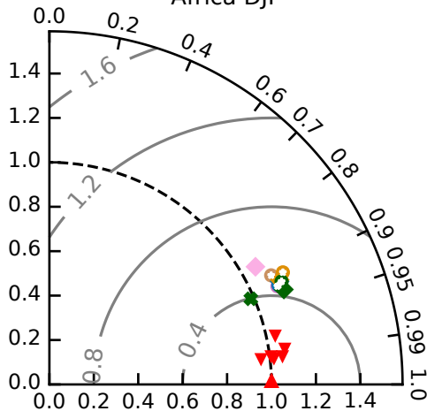
Africa DJF
