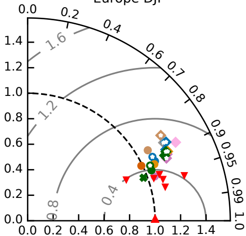
Europe DJF
