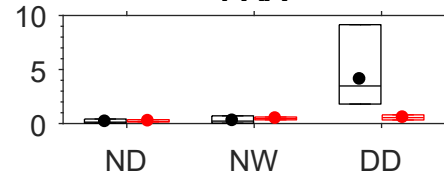
HPALD
