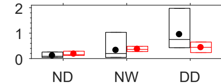
DHC 4
