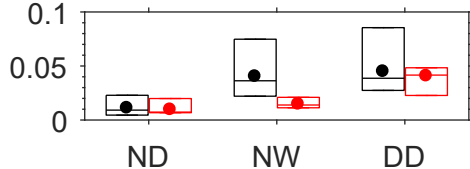
HCN
