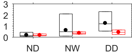
HCN
