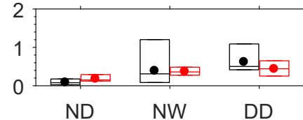
MTNP
