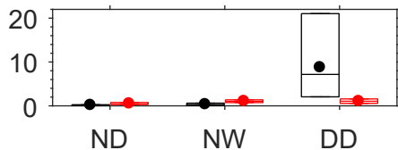
HDC 4
