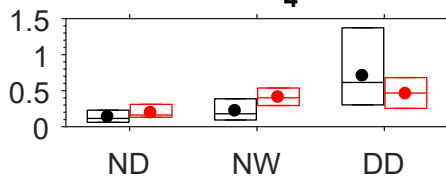
PROPNN
