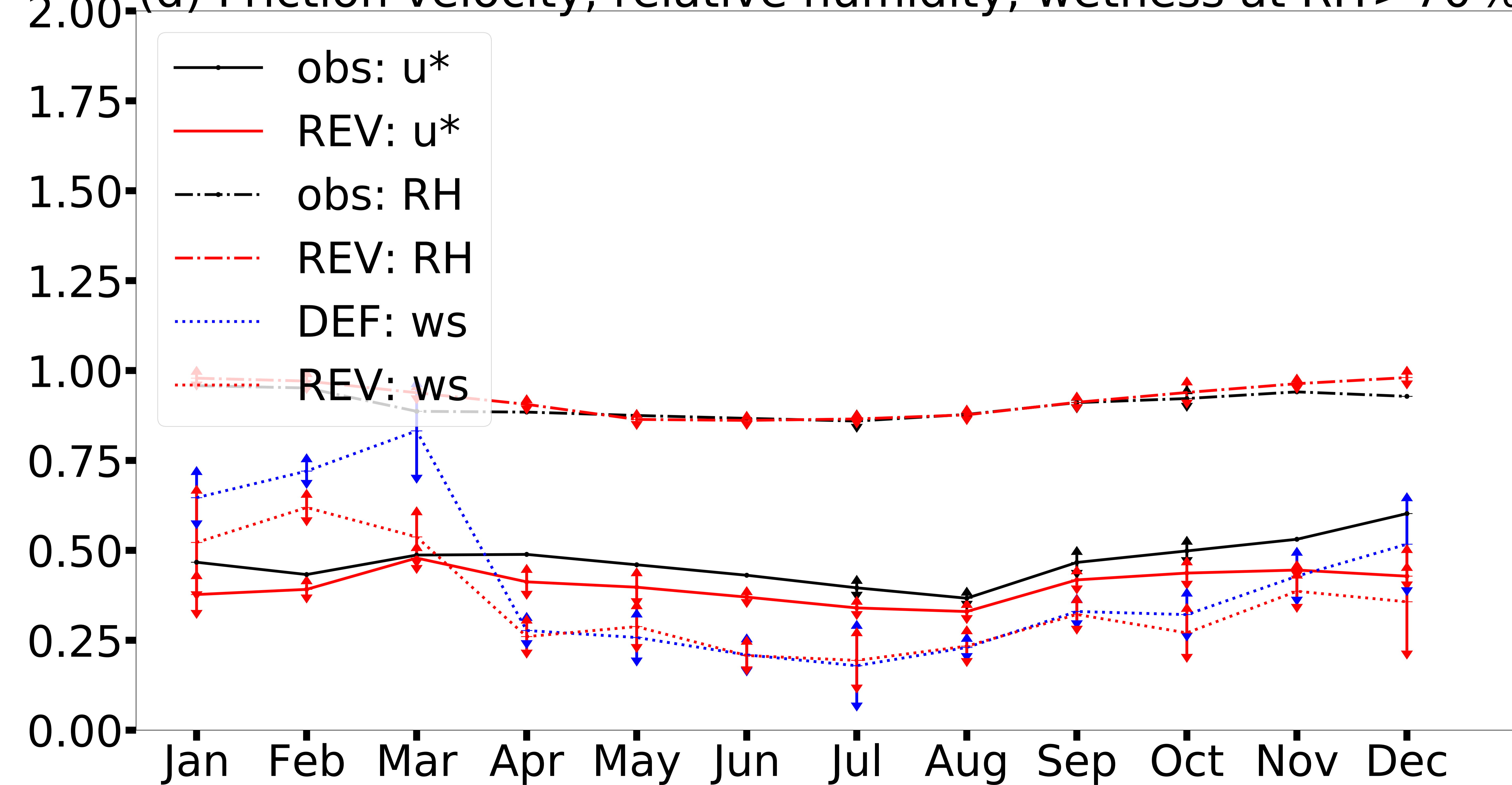
(d) Friction velocity, relative humidity, wetness at RH &gt; 70 %
