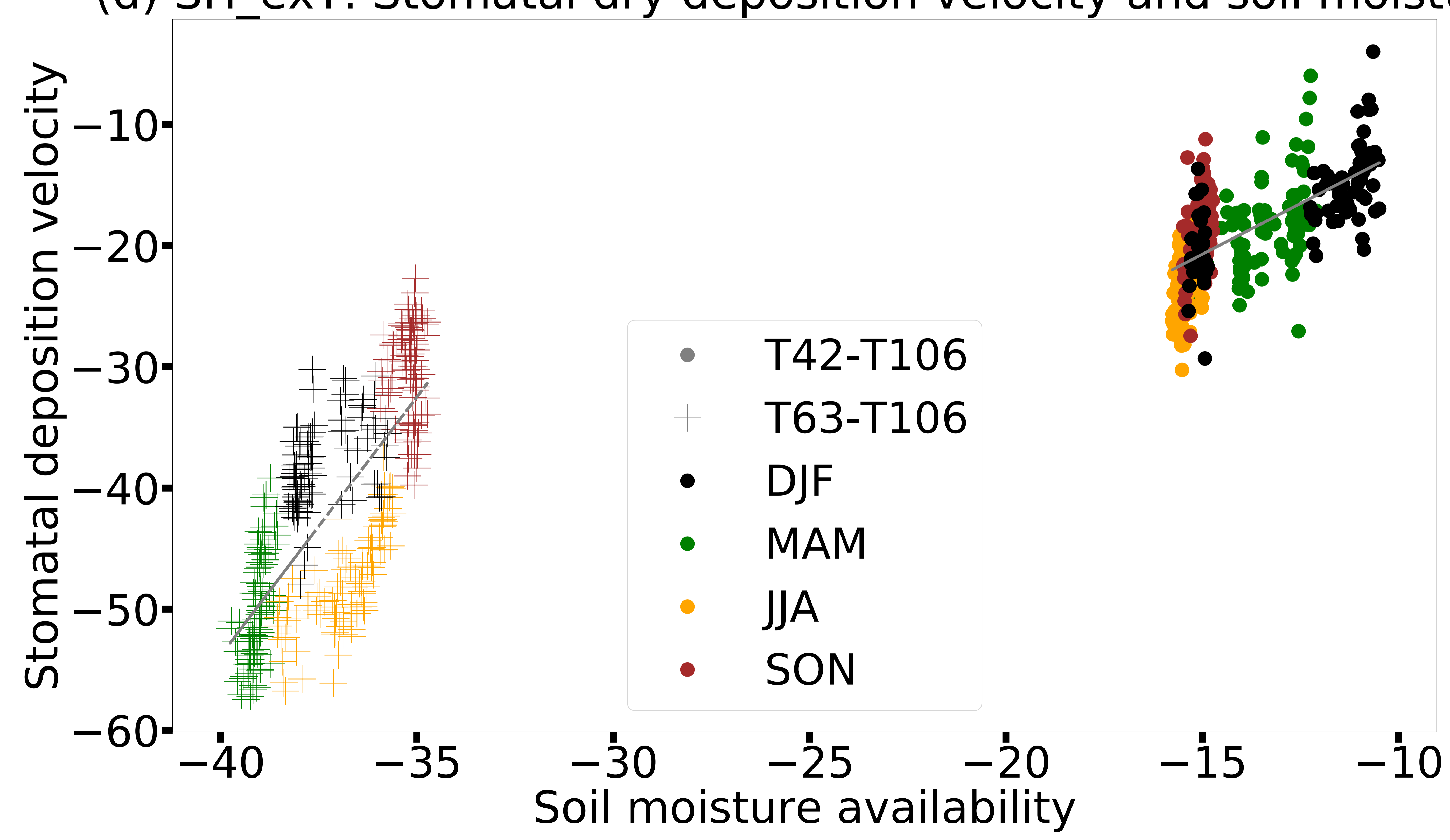
(d) SH_exT: Stomatal dry deposition velocity and soil moisture
