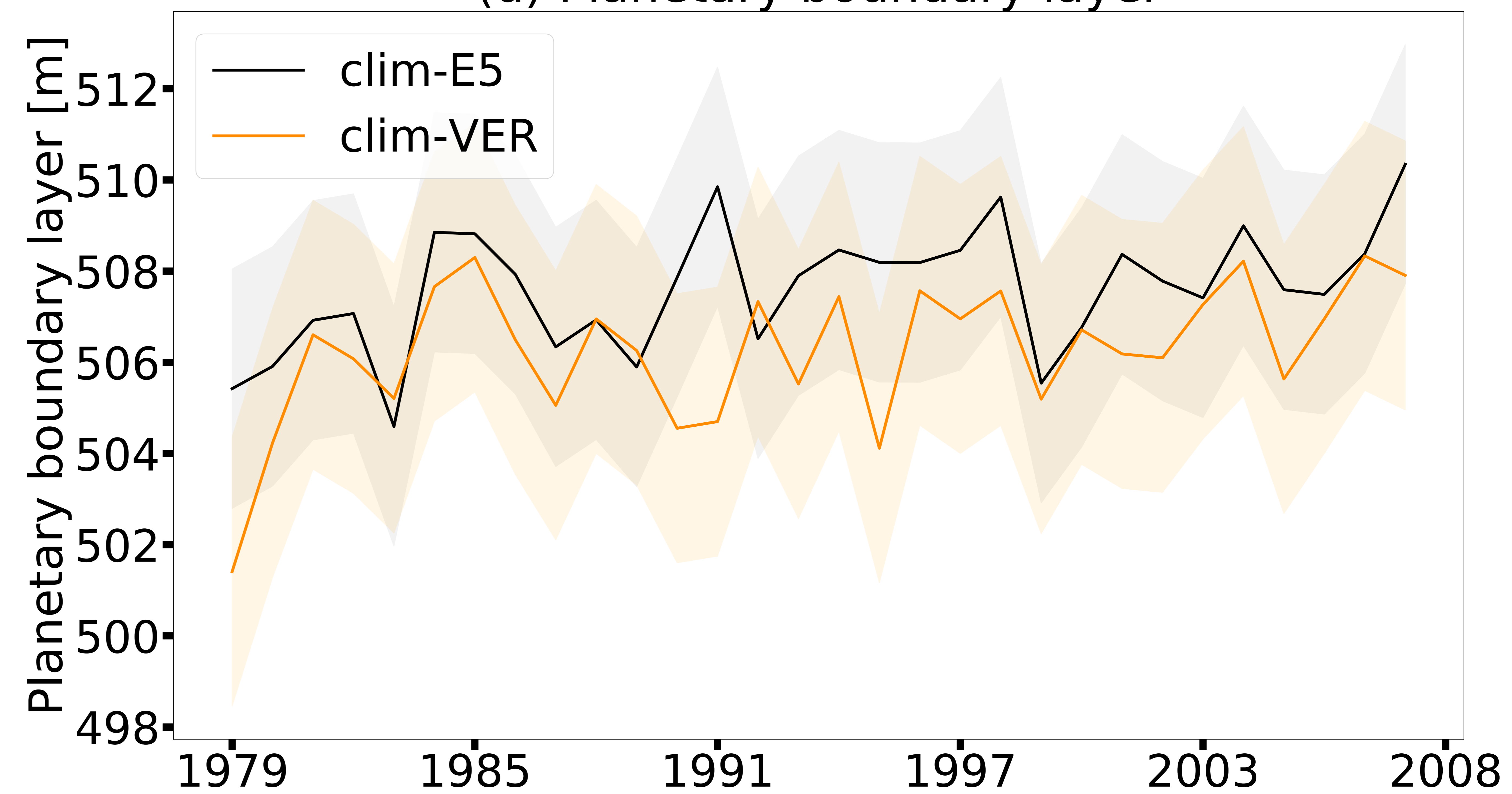
(d) Planetary boundary layer
