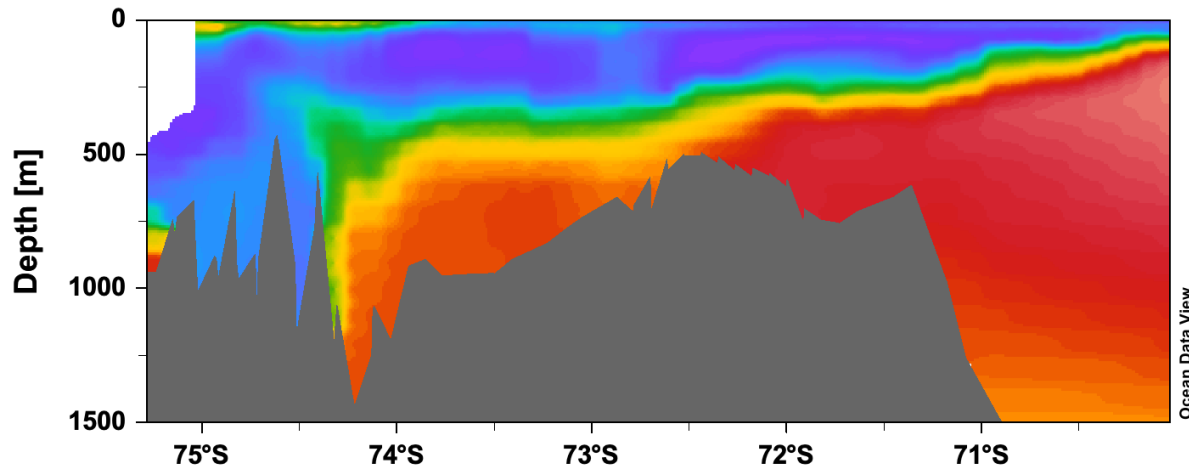
(a) 2014 Pot. Temp., iter0
