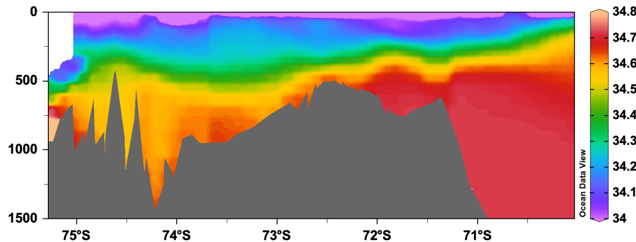
(d) 2014 Salinity, iter20
