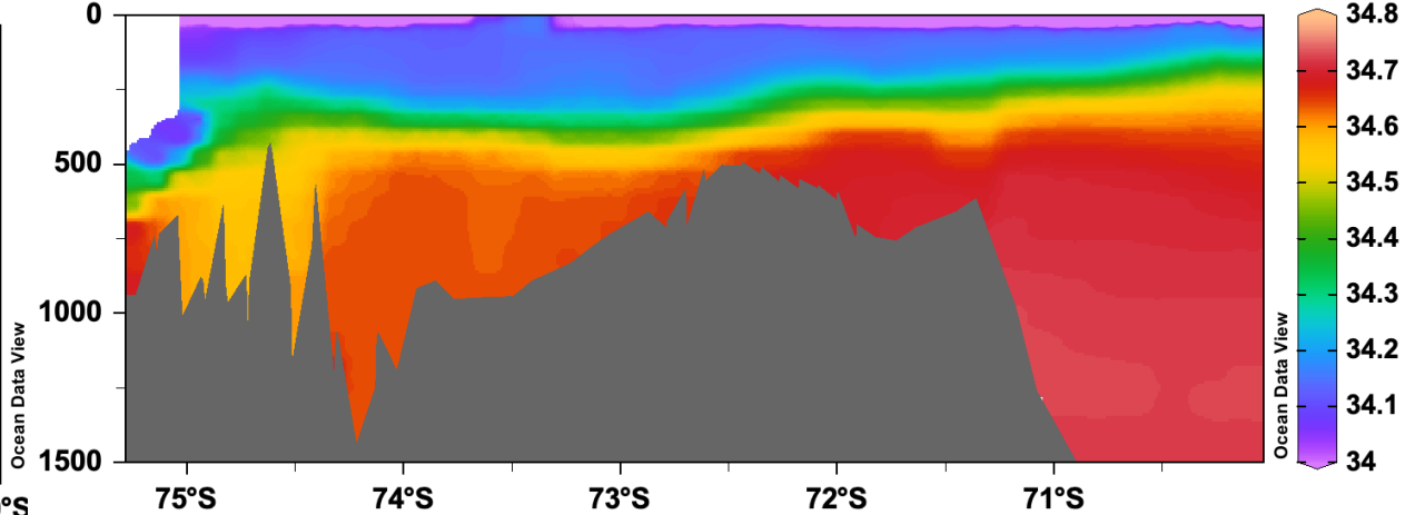
(d) 2010 Salinity, iter20
