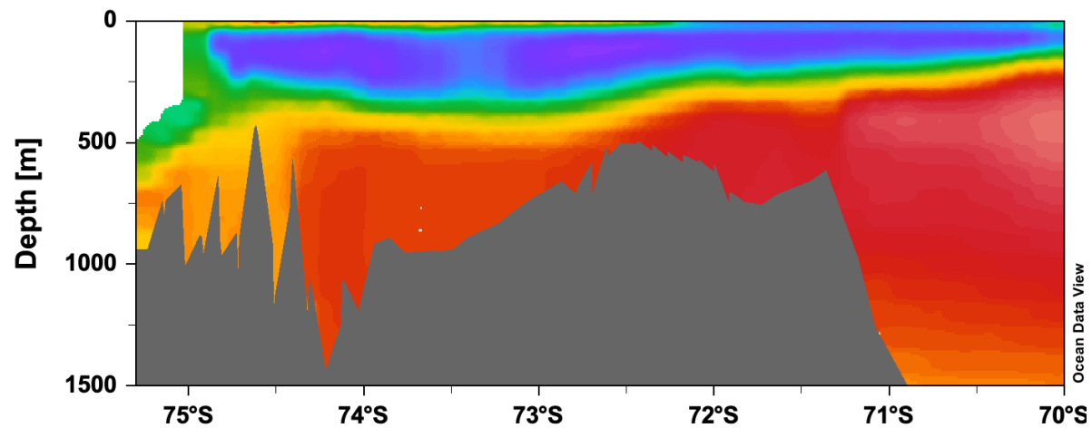
(a) 2010 Pot. Temp., iter0
