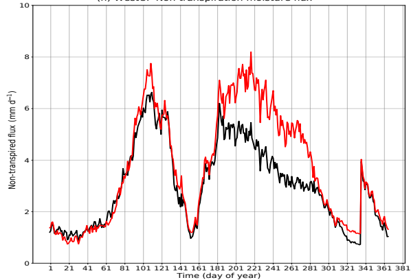
(h) WestUP Non transpiration moisture flux
