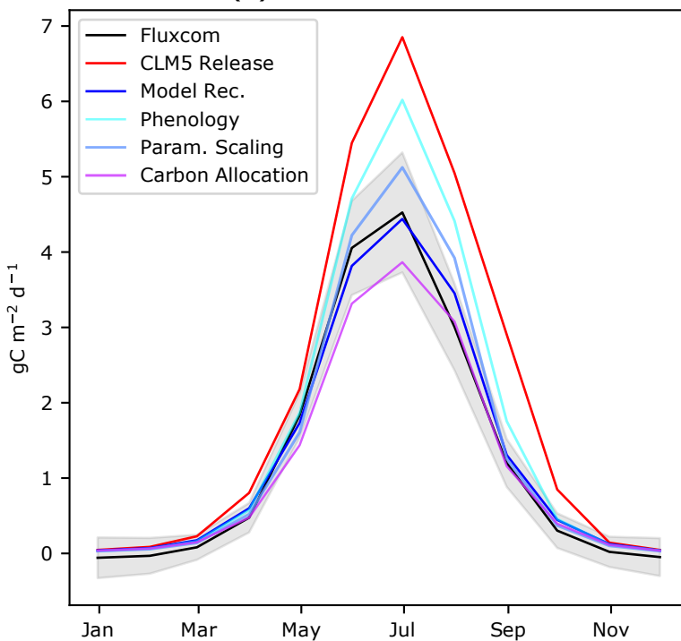
(d) BDT GPP
