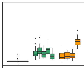
LSTM(All variables, 95)
