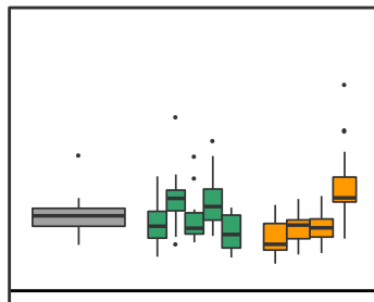
MLP(All variables)
