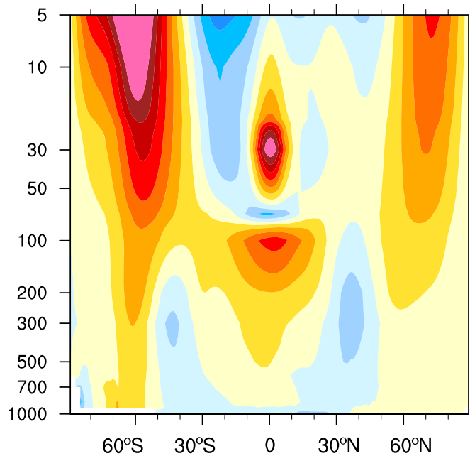
(d) BCC-CSM2-HR minus ERA5 U
