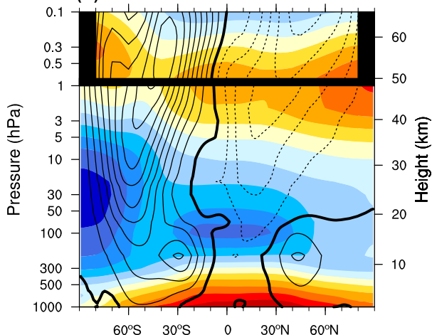
(d) BCC-CSM2-MR
