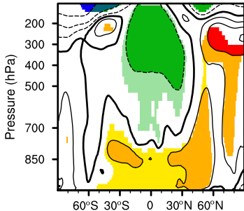
(d) \Delta Q ( \text{g kg}^{-1} )
