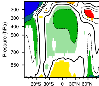
(e) \Delta Q ( \text{g kg}^{-1} )
