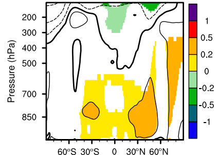
(f) \Delta Q ( \text{g kg}^{-1} )
