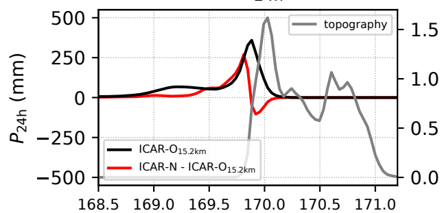
(h) P_{24h}
