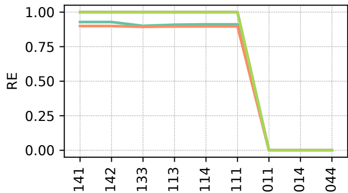
(d) \bar{q}_{\text{prc}}
