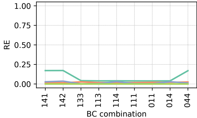
(d) \bar{q}_{\text{prc}}
