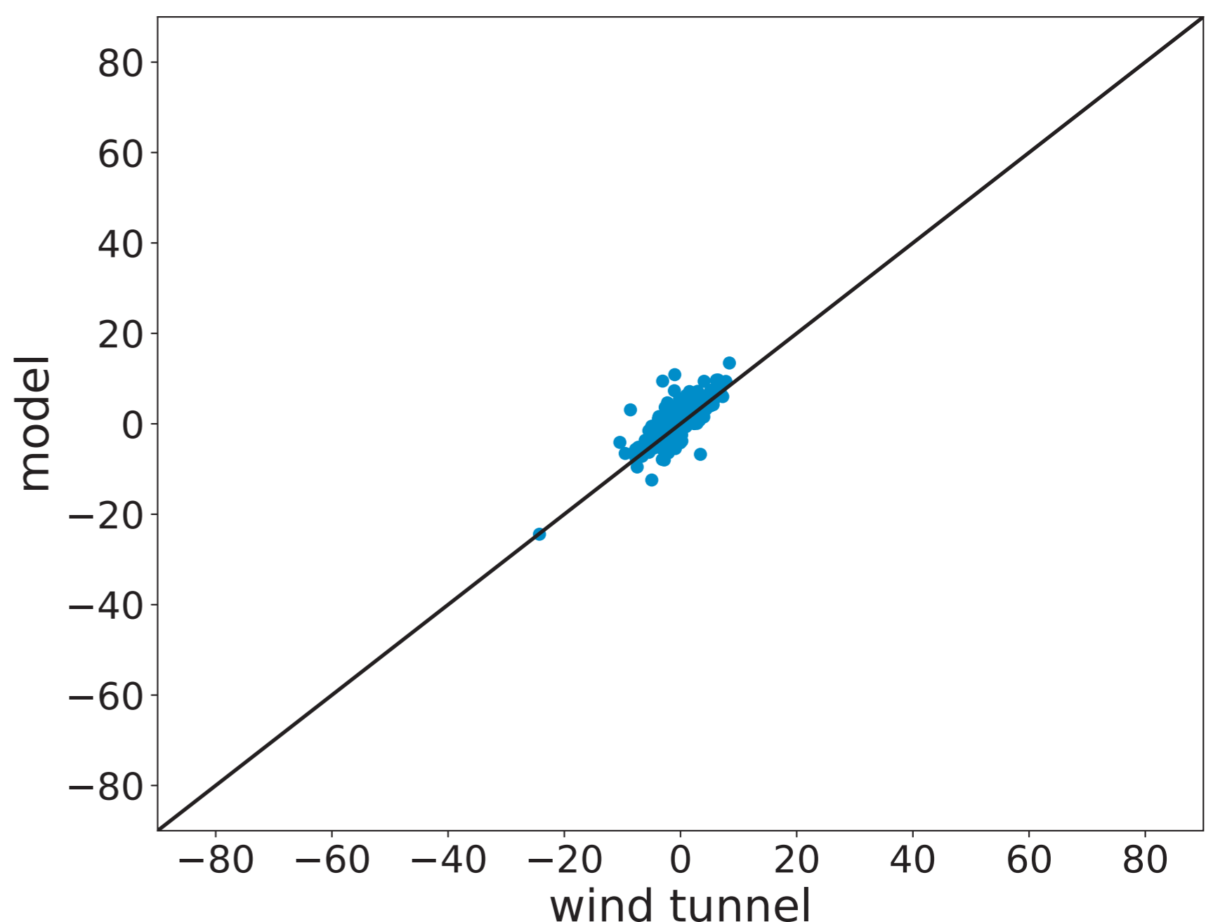
(d) Horizontal wind direction \arctan(v/u) 27 m [°]
