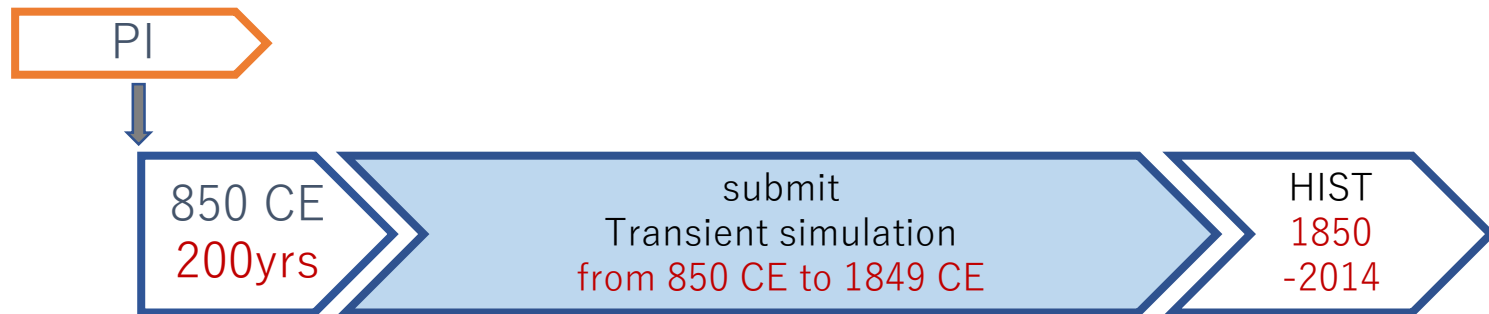
(d) Spin-up procedure of LM and HIST
