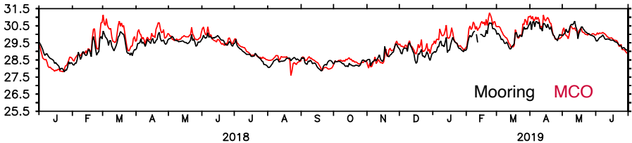
(b) SST M_2(8^\circ \text{ S}, 95^\circ \text{ E})
