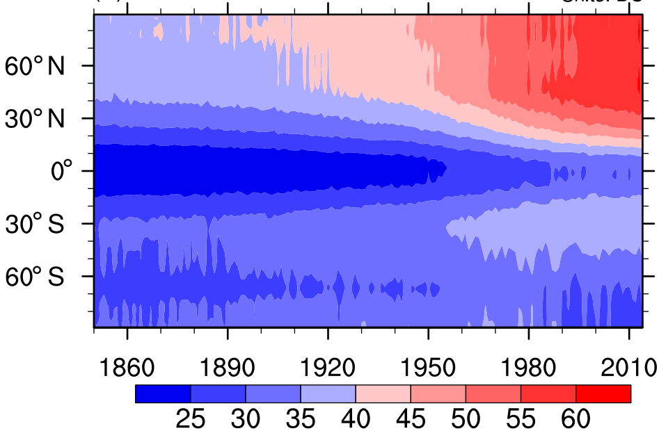
(b) CMIP6
