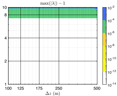
(d) M2b
