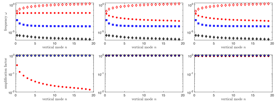
(d) Spacetime operator for M2be
