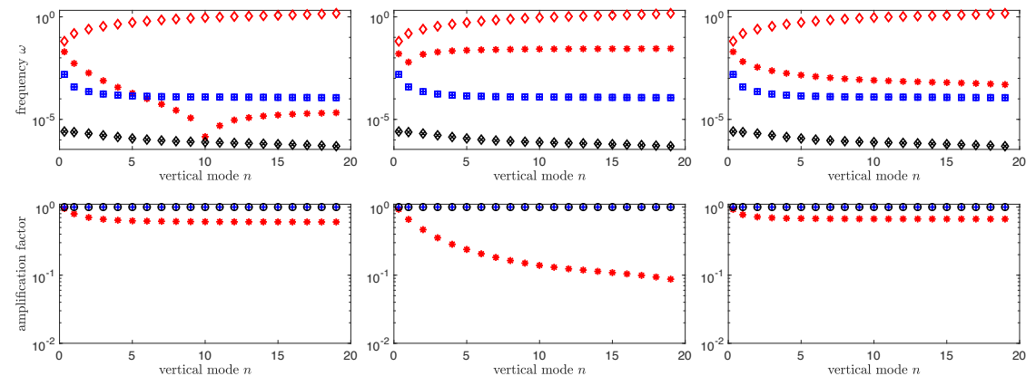
(d) Spacetime operator for M2a
